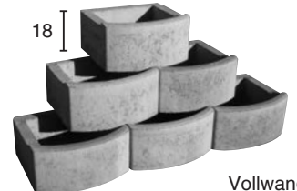
Vollwand
